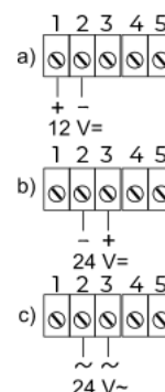
Rysunek 2 Podłączenie zasilania
