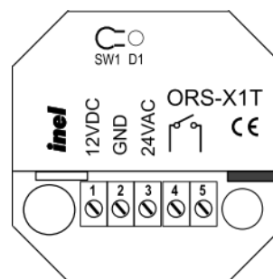
Rysunek 1 Widok odbiornika
